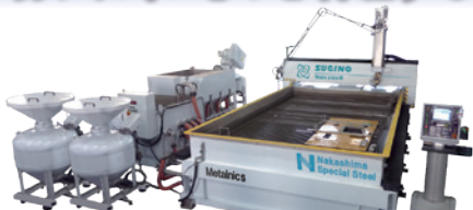
(Made In Japan) アプレシブジェットカッタ NC-5AX 2キ/マシン製
